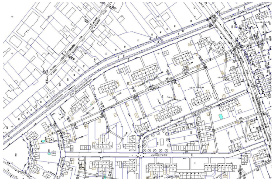
Ausschnitt Kanalverlauf Altsiedlung
